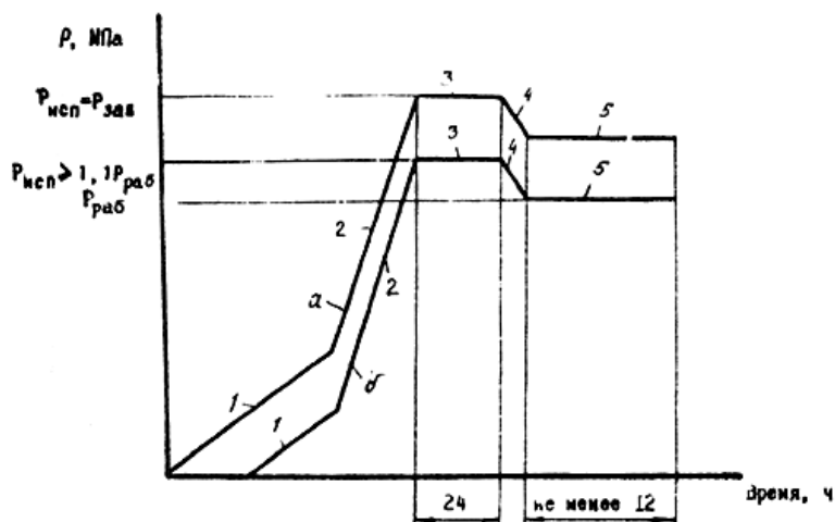
Рис.10. График изменения давления при гидравлическом испытании магистральных нефтепроводов и нефтепродуктопроводов:
