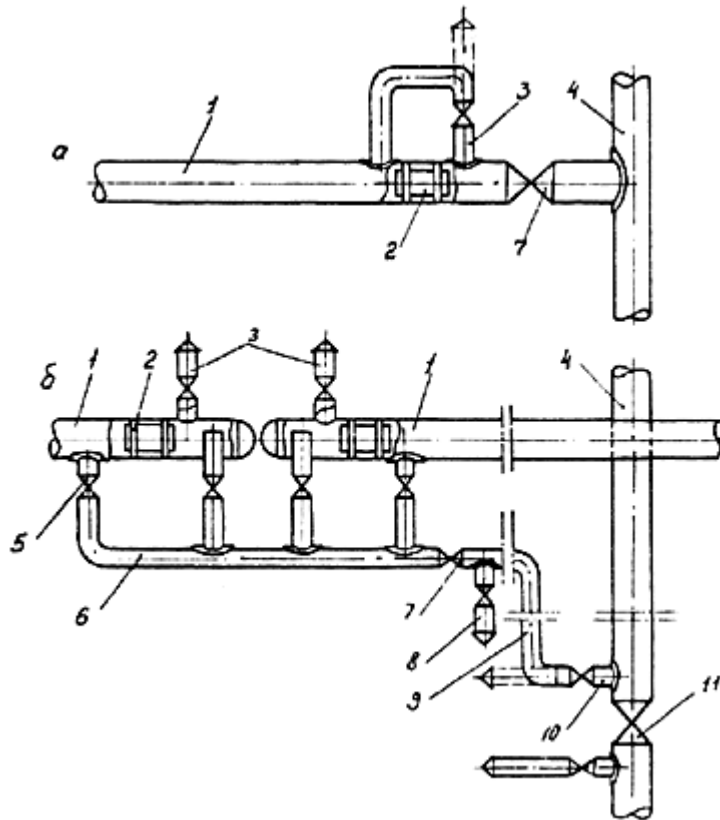
Рис.5. Принципиальная схема подключения для отбора природного газа из действующих газопроводов:
