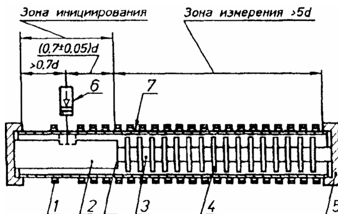
1 - кольца наружной обоймы; 2 - наковальня; 3 - несущий стержень; 4 - декомпрессионные перегородки; 5 - заглушки; 6 - боек; 7 - испытуемый образец Рисунок 2
