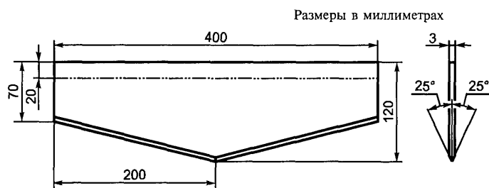
Рисунок 7 — Стальное лезвие для иницирования трещины в полиэтиленовой трубе
