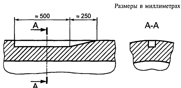
Рисунок 6 — Канавка, обрабатываемая на наружной поверхности трубы
