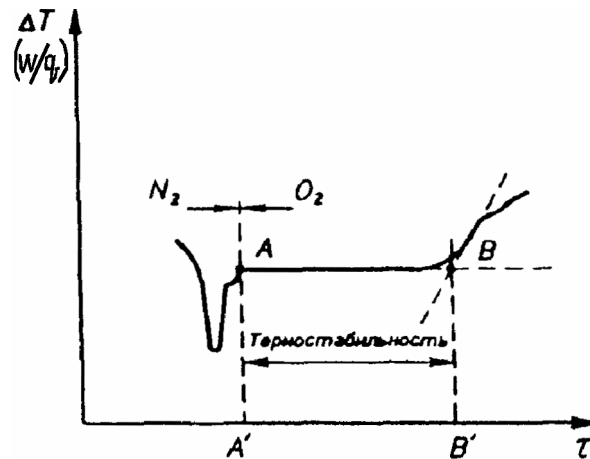
Рисунок 1 - Типичная кривая окислительной термостабильности полиэтилена
